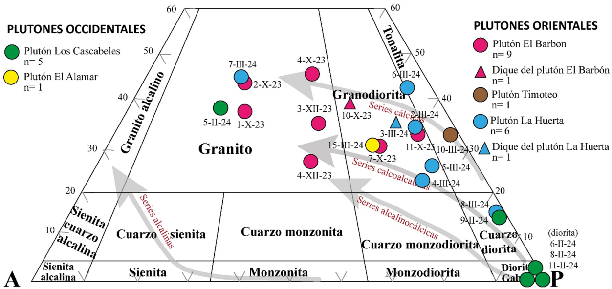
Figura 6. Diagrama de clasificación modal QAP (Le Maitre et al., 2002) de las rocas intrusivas del Valle Ojos Negros y series composicionales para rocas plutónicas según Frost y Frost (2008).
