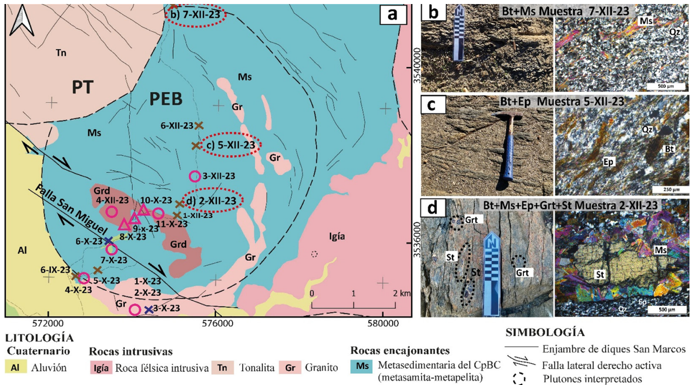
Figura 4. a) Mapa geológico de la zona del plutón El Barbón. Las muestras de las rocas encajonantes meta-sedimentarias del Complejo Bedford Canyon (Ms) analizadas petrográficamente están en cruces. b) En la izquierda, afloramiento de metasamitas de grano medio y a la derecha la lámina delgada correspondiente que muestra textura lepidoblástica, con clivaje de crenulación marcado por cristales de muscovita. c) En la izquierda, afloramiento de metapelita con foliación definida por biotita y muscovita; en lámina delgada se reconocen planos de cizalla con biotita intercalada y epidota alojada en planos de deformación. d) En la izquierda afloramiento de metapelita-samita de grano fino con granate y estaurolita resaltada en líneas discontinuas. Abreviaturas: Bt: Biotita, Ep: Epidota, Grt: Granate, Ms: Muscovita, Qz: Cuarzo y St: Estaurolita.
