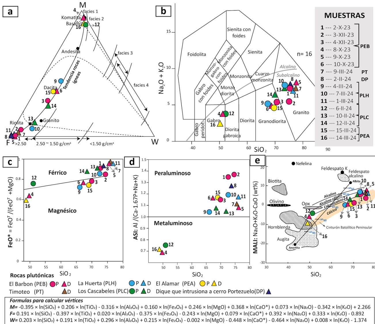
Figura 12. Diagramas de clasificación geoquímica para las rocas plutónicas del Valle Ojos Negros. a) Diagrama de índice de Intemperismo químico MFW de Otha y Arai (2007), donde M, F y W representan las fuentes máficas, félsicas y materiales intemperizados, respectivamente. Las líneas discontinuas en (a) representan tendencias lineales composicionales para los perfiles de meteorización de basalto, diorita y granito, b) Diagrama de álcalis total vs. sílice (TAS; Middlemost 1994) de las rocas intrusivas, con la subdivisión entre las series alcalina y subalcalina de Irvine y Baragar (1971; tomado de Rollinson y Pease, 2021). c) Diagrama de sílice vs. \text{FeO}^* = \text{FeOT}/(\text{FeOT}+\text{MgO}) , d) Diagrama de sílice vs. índice de saturación de aluminio (ASI) y e) Diagrama de sílice vs. índice modificado de álcalis menos CaO (MALI) donde se muestra que la mayor parte de las muestras se encuentran en el campo cálcico, que caracteriza al Cinturón Batolítico Peninsular. El listado numérico indica la clave de cada muestra. Abreviaturas: PEB: plutón El Barbón, PT: plutón Timoteo, DP: dique en el cerro El Portezuelo, PLH: plutón La Huerta, PLC: plutón Los Cascabeles, pEA: Plutón El Alamar.
