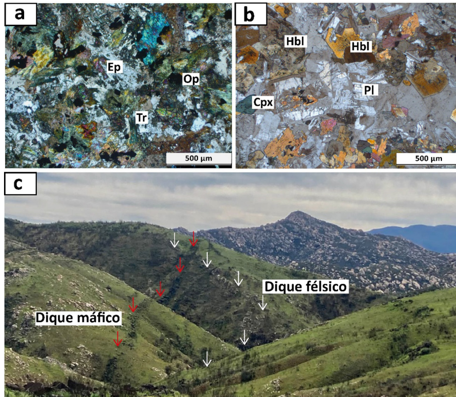
Figura 9. a) Microfotografía de diorita de hornblenda tremolitizada con hábitos fibrosos, b) Microfotografía de cuarzodiorita de hornblenda, c) Diques asociados al enjambre de diques San Marcos (señados con flechas rojas) expuestos en el sector del plutón Los Cascabeles. Los diques félsicos marcados con flechas blancas son más jóvenes y cortan a los de San Marcos. Abreviaturas: Cpx: Clinopiroxeno, Ep: Epidota, Hbl: Hornblenda, Op: Opacos, Pl: Plagioclase y Tr: Tremolita.
