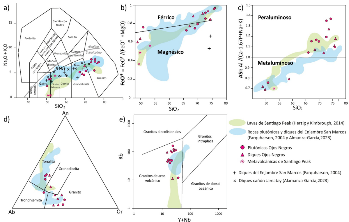
Figura 16. Diagramas de clasificación geoquímica de las rocas ígneas del Valle Ojos Negros, marcadas con símbolos en color rosa (este trabajo). Conjunto de muestras de la Formación Santiago Peak en el campo color verde (Herzig y Kimbrough, 2014) y conjunto de diques del Enjambre San Marcos en el campo azul (Farquharson, 2004 y Almanza-García, 2023). a) Diagrama de álcalis totales vs. sílice (TAS; Middlemost, 1994) para rocas plutónicas. b) Diagrama de sílice vs. \text{FeO}^* (Frost y Frost, 2008). c) Diagrama de sílice vs. índice de saturación de aluminio (ASI; Frost y Frost, 2008). d) Diagrama de clasificación An-Ab-Or (Barker, 1979) para rocas graníticas de acuerdo con su composición normativa CIPW. e) Diagrama de discriminación tectónica para granitos Y+Nb vs Rb (Pearce et al., 1984).
