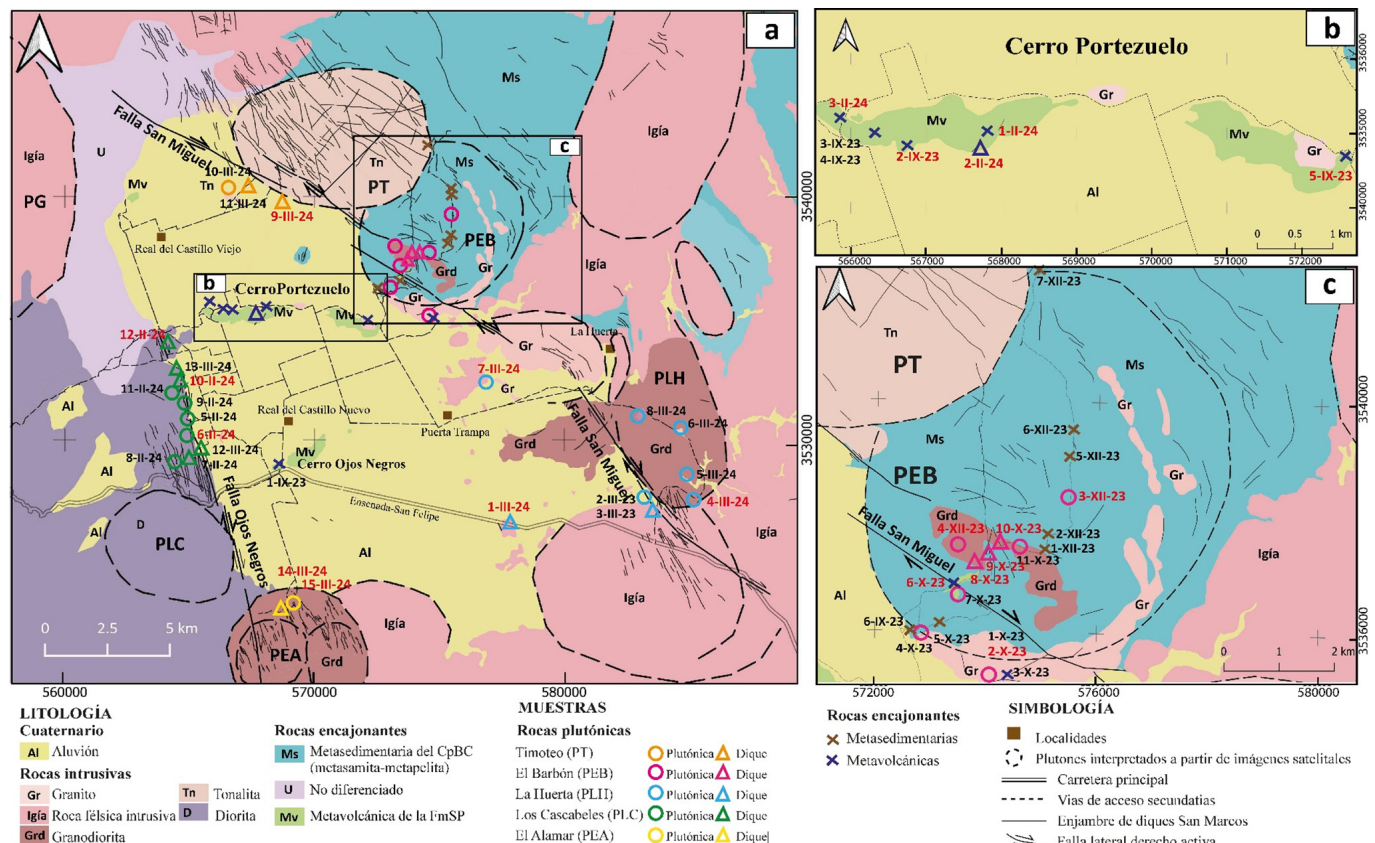
Figura 2. Mapa geológico de la región del Valle Ojos Negros y distribución de muestras analizadas petrográficamente en negro y geoquímicamente en color rojo. a) Distribución de los plutones Timoteo, El Barbón, La Huerta, Los Cascabeles y El Alamar interpretados a partir de imágenes satelitales. b) Rocas volcánicas de la Fm. Santiago Peak en el cerro Portezuelo. c) Rocas encajonantes metasedimentarias asociadas con el Complejo Bedford Canyon en la zona del plutón El Barbón. Base cartográfica tomada de las cartas: H11B12, H11B13, I11D83 y I11D84 del INEGI (1976a; 1976b; 1977a; 1977b) y del mapa de reconocimiento geológico de Gastil et al. (1975). Abreviaturas: PEA: Plutón El Alamar, PEB: Plutón El Barbón, PG: Plutón Guadalupe, PLC: Plutón Los Cascabeles, PLH: Plutón La Huerta, PT: Plutón Timoteo. Sistema de coordenadas geográficas: WGS 84/ UTM zona 11.
