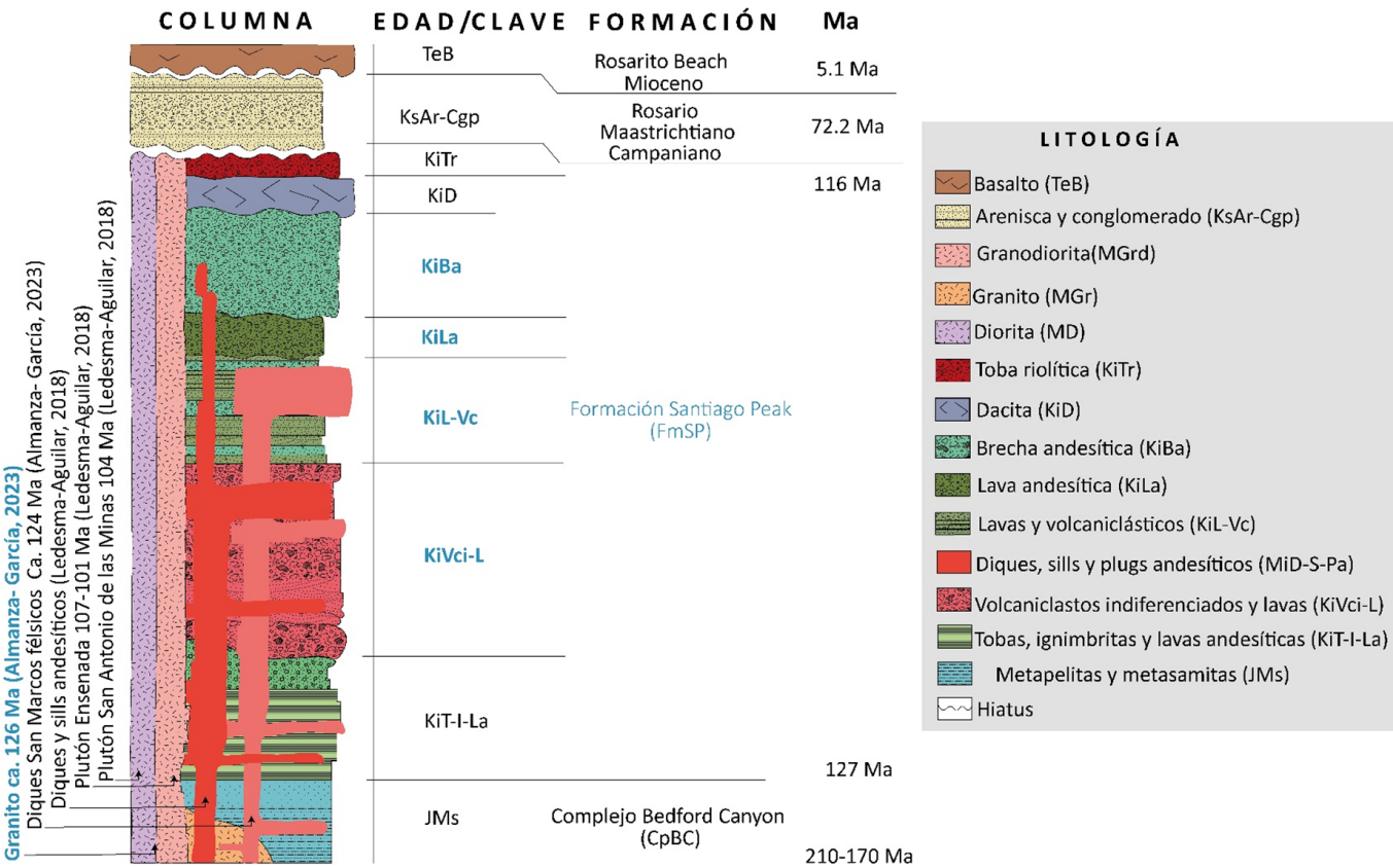
Figura 3. Columna estratigráfica compuesta de la litología que aflora entre Ensenada y Valle Ojos Negros (modificada de Ledesma-Aguilar, 2018). En color azul se muestran las unidades que afloran en el área de Ojos Negros y en negro las expuestas en Ensenada.
