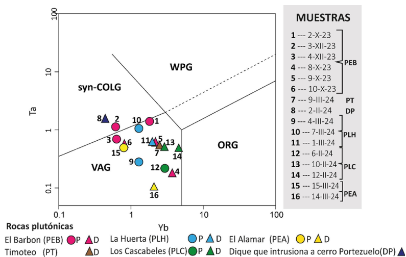
Figura 15. Diagrama de discriminación tectónica para granitos (Pearce et al., 1984). Abreviaturas: VAG: granitos de arco volcánico, syn-COLG: granitos sincollisionales, WPG: granitos intraplaca and ORG: granitos de dorsal oceánica (ORG).
