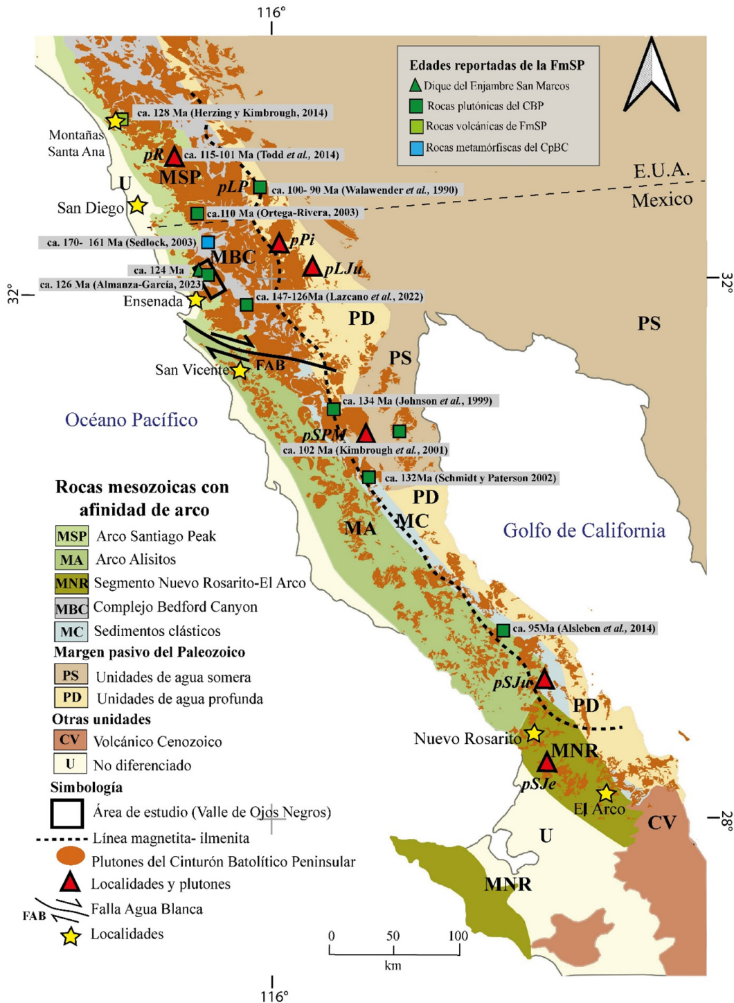
Figura 1. Mapa de la región del Cinturón Batolítico Peninsular (CBP). Las provincias tectonoestratigráficas prebatolíticas están definidas por sus afinidades litológicas y geocronológicas (Modificado de Contreras-López et al., 2021). La línea discontinua de color negro es la línea magnetita-ilmenita de Gastil et al. (1990). En la porción norte del CBP, en el SW de E.U.A. se indica el complejo plutónico Ramona (PR; Todd et al. , 2014), el cual es comparable con los plutones del Valle Ojos Negros, en el rectángulo negro. Las edades U-Pb en círculo se obtuvieron de rocas metamórficas prebatolíticas (Complejo Bedford Canyon y Formación Santiago Peak), rocas plutónicas y diques del Enjambre San Marcos.
