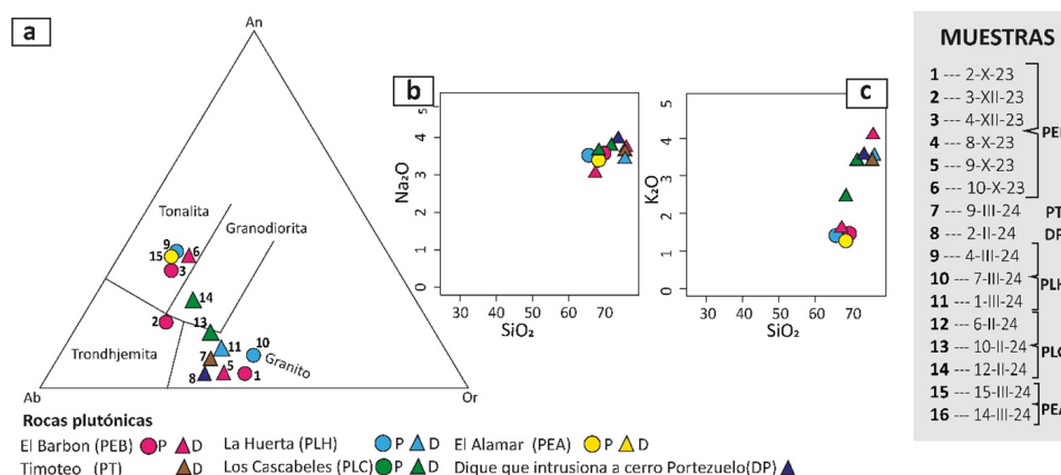
Figura 13. a) Diagrama de clasificación An-Ab-Or normativos de Barker, (1979). b) Diagrama Na 2 O vs. sílice. c) Diagrama K 2 O vs. sílice.
