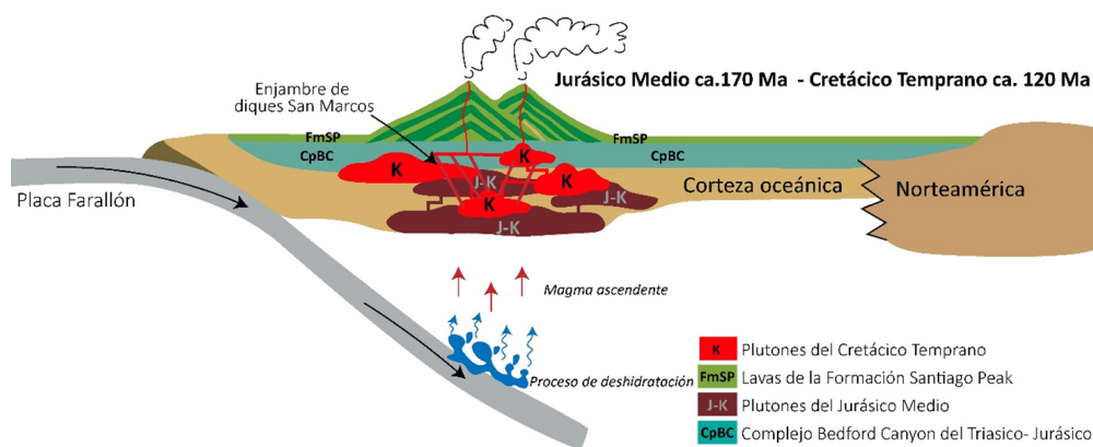
Figura 17. Modelo tectónico esquemático que ilustra la evolución magmática y tectónica del sur de California, E.U.A. y noroeste de Baja California en donde estaría la región del Valle Ojos Negros. Durante el Triásico al Jurásico Medio debieron depositarse las rocas sedimentarias con material derivado del continente del Complejo Bedford Canyon, el cual está sobreyacido por rocas volcánicas del segmento de arco Santiago Peak del Jurásico-Cretácico Temprano cerca del margen continental y que representan el extremo norte del Cinturón Batolítico Peninsular. El magmatismo de arco fue continuo hasta el Cretácico Temprano. Los plutones más jóvenes intrusionan al basamento y a las rocas más antiguas del arco, representadas por las sucesiones volcánicas de la Formación Santiago Peak.
