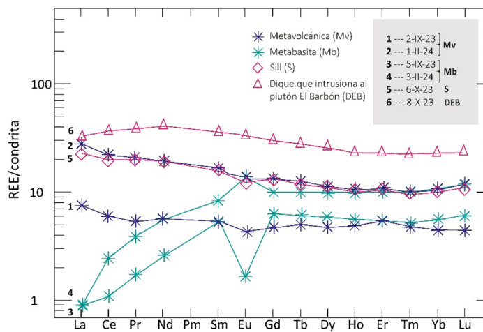
Figura 11. Diagrama de elementos de tierras raras normalizados a condrita (McDonough y Sun, 1995) para las rocas metaígneas del Valle Ojos Negros pertenecientes a la Formación Santiago Peak.
