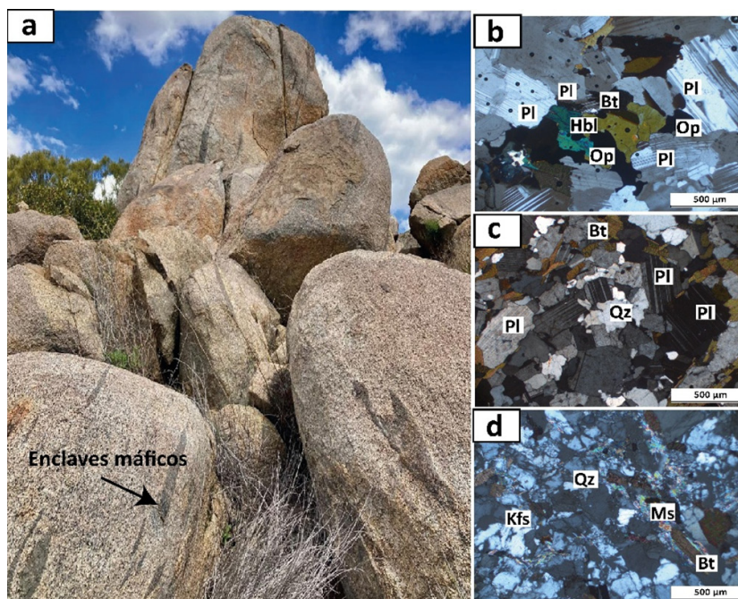
Figura 8. a) Afloramiento de cuarzodiorita del plutón La Huerta con enclaves máficos elongados paralelos a la foliación. b) Microfotografía de cuarzodiorita de hornblenda y biotita con plagioclasa (oligoclase-andesina), c) Microfotografía de granodiorita de biotita de grano medio, d) Microfotografía de granito de dos micas de grano fino a medio fuertemente fracturada. Abreviaturas: Bt: Biotita, Hbl: Hornblenda, Kfs: Feldespato potásico, Ms: Muscovita, Op: Opacos, Pl: Plagioclasa y Qz: Cuarzo.
