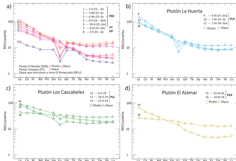
Figura 14. Diagrama de elementos de tierras raras normalizados a condrita (McDonough y Sun, 1995) para las rocas plutónicas y diques del área de estudio, separada por plutón analizado.
