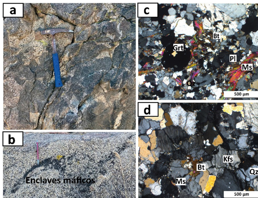
Figura 7. a) Mingling de diorita en tonalita b) Enclaves máficos plegados dentro de un cuerpo granítico. c) Microfotografía de un granito con textura hipidiomórfica de dos micas con granate (Grt). d) Microfotografía de un granito de dos micas con texturas de exsolución en feldespatos potásicos. Abreviaturas: Bt: Biotita, Grt: Granate, Kfs: Feldespato potásico, Ms: Muscovita, Pl: Plagioclasa y Qz: Cuarzo. plutónicas según Frost y Frost (2008).
