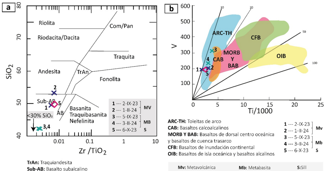
Figura 10. Clasificación geoquímica de las rocas metaígneas del Valle Ojos Negros. a) Diagrama \text{SiO}_2 vs. \text{Zr}/\text{TiO}_2 (Winchester y Floyd, 1977). b) Clasificación tectonomagmática de rocas basálticas \text{Ti}/1000 vs. V (Shervais, 1982).
